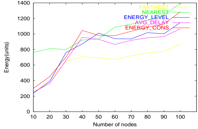
Fig. 10. Energy per message
